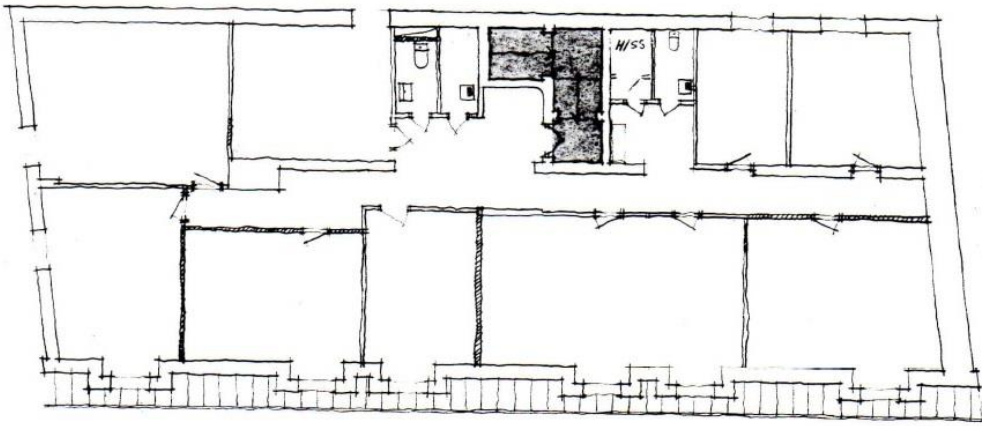
PLATT, VÄNING 2 TRAPPOR SKALA 1:100
