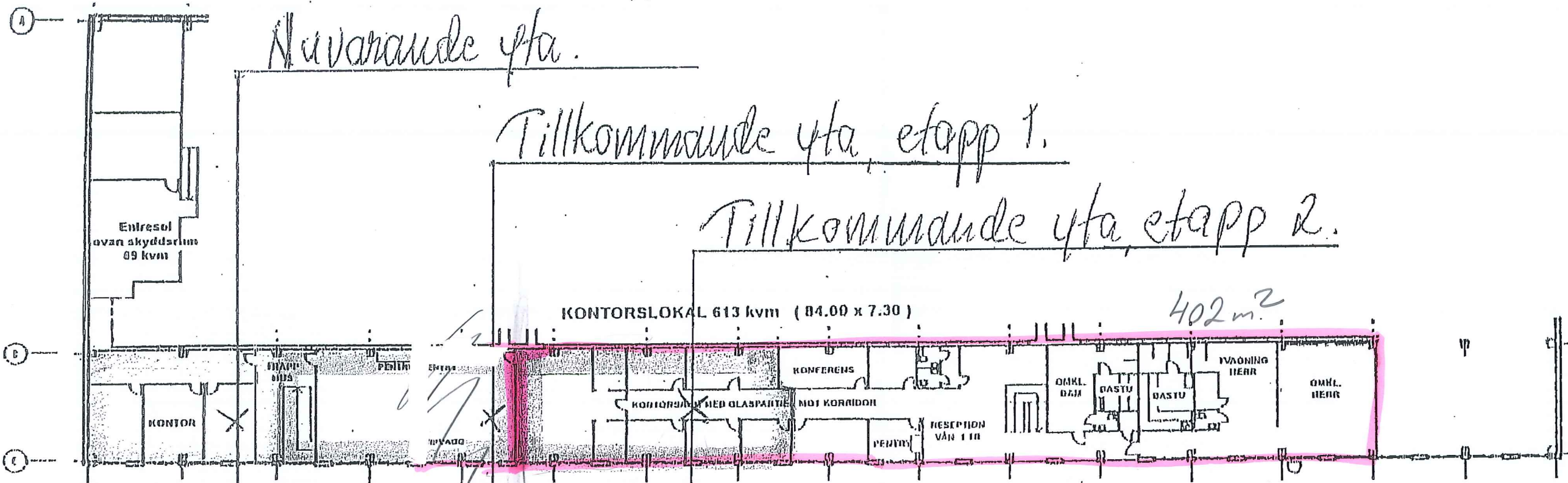
PLAN ENTRESOL
