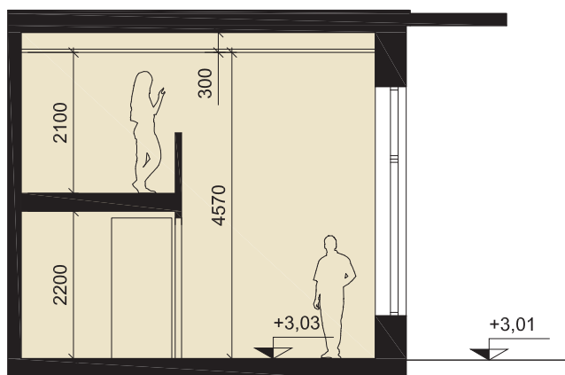
SEKTION
