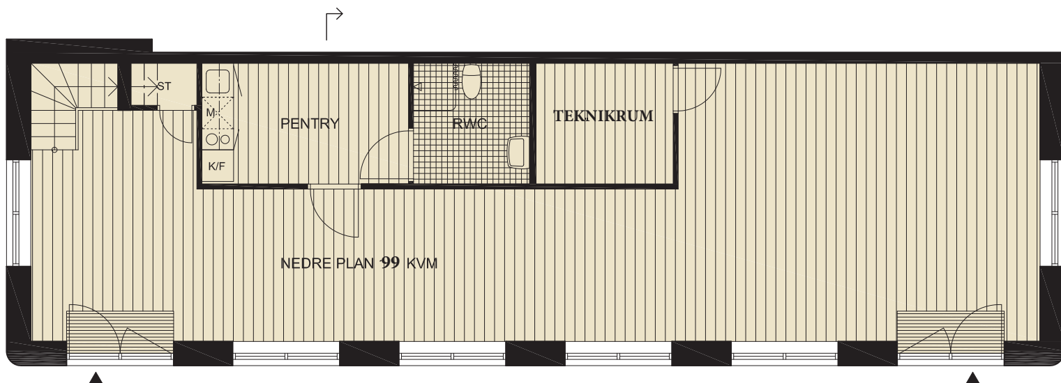
ENTRÉPLAN
