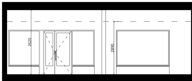
SEKTION A-A
