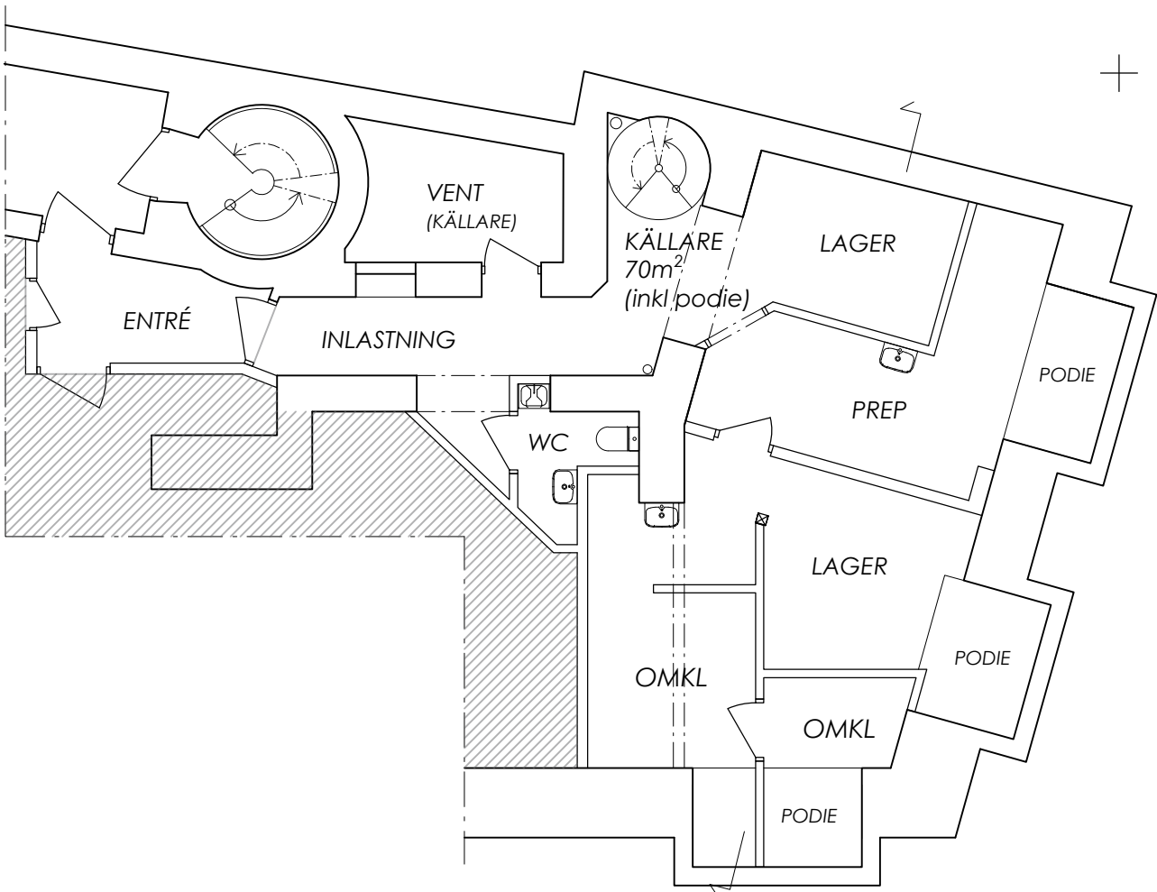
KÄLLARVÅNING SKALA 1:100
