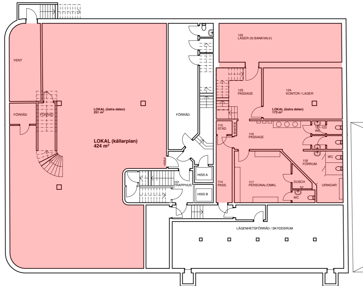
KÄLLARPLAN Skala 1:200
