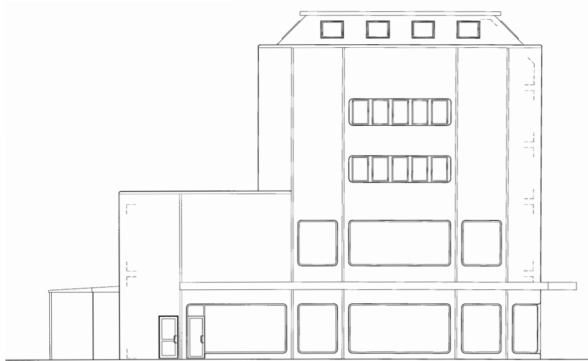
FASAD MOT VÄSTER (MAGASINSGATAN) Skala 1:200
