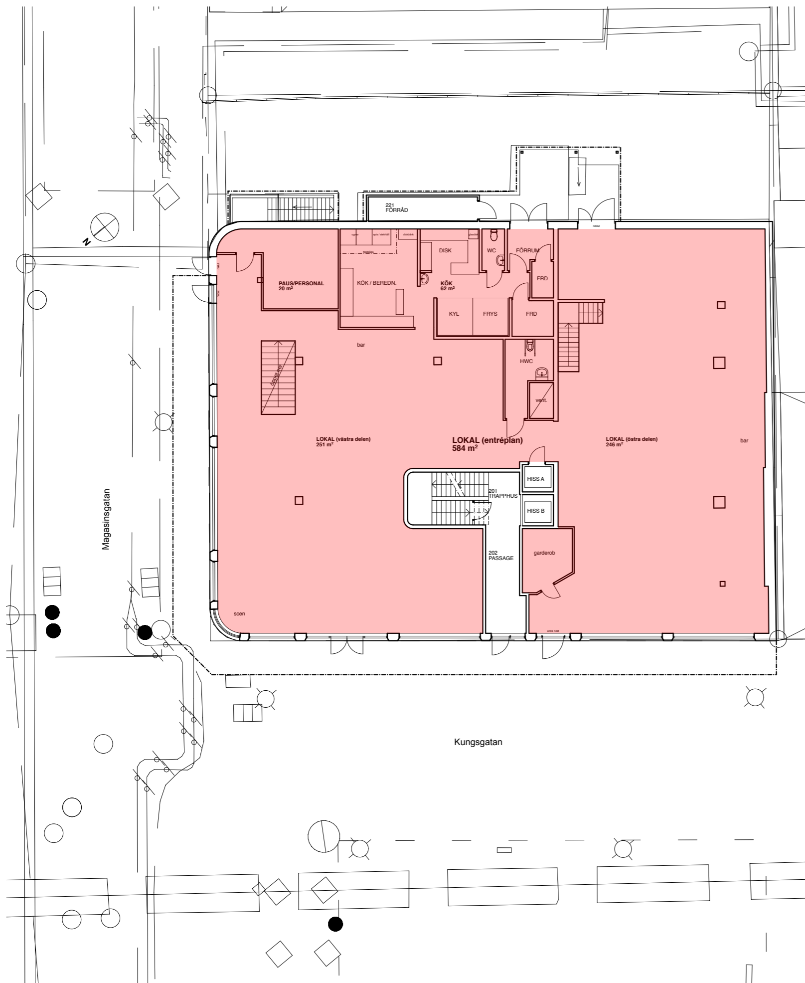
ENTRÉPLAN Skala 1:200
