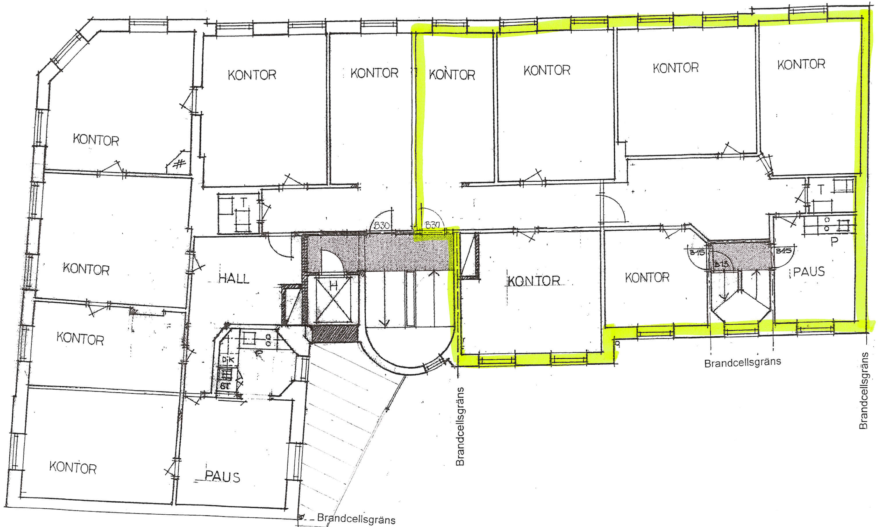
Våningsplan 1 trappa sk. 1:100
