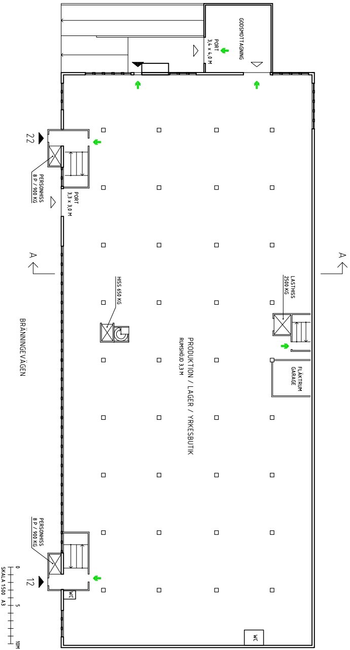
PLAN 2, ENTRÉVÅNING
