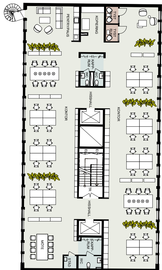
PLAN 6, CA 370 KVM KONTOR FÖR CA 35-40 PERSONER
