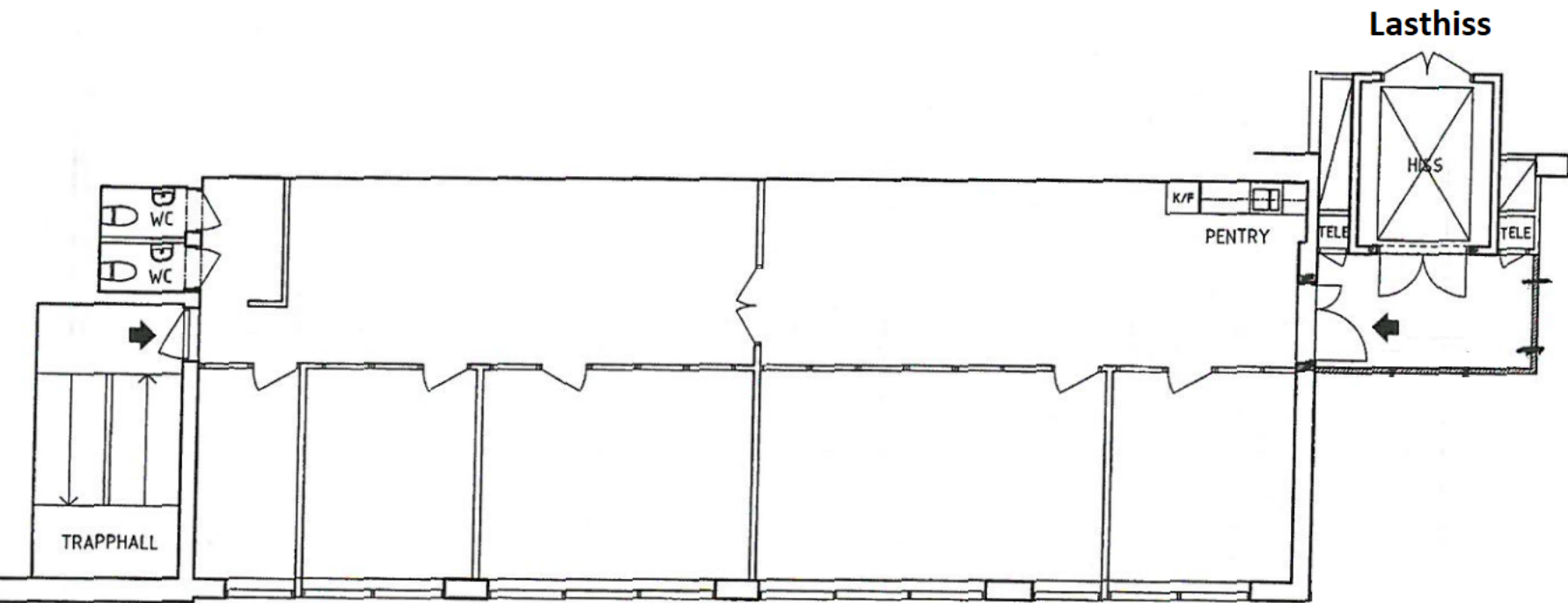
KONTORSLOKAL PLAN 03 - VÅN 1 TR LOA 155 m 2
