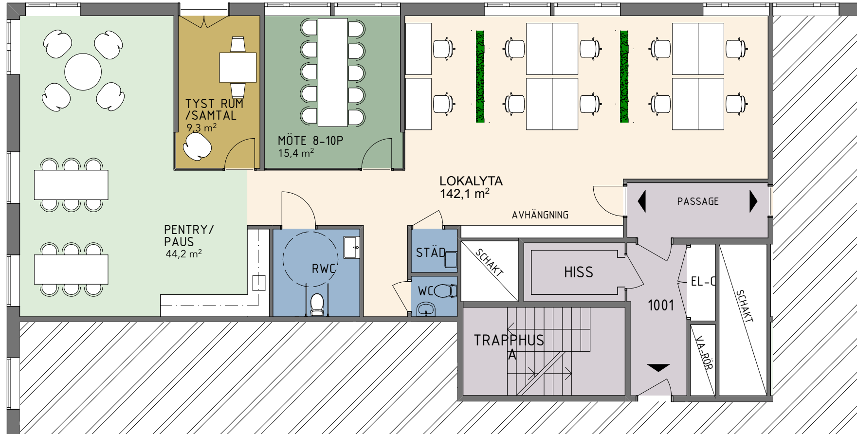
PLAN 2, 1TR SKALA 1:100/ A3
